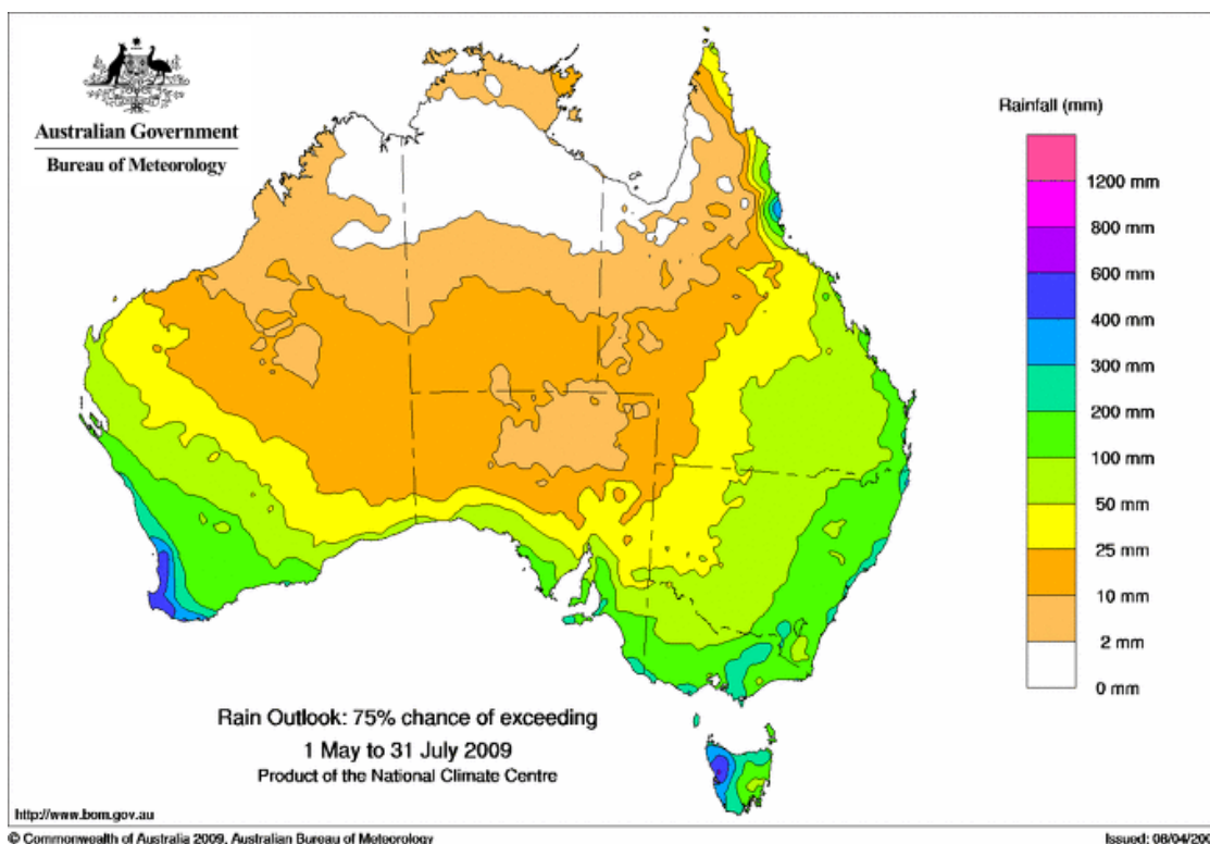
豪州 5/1から7月末までの降雨予想 豪州気象局
