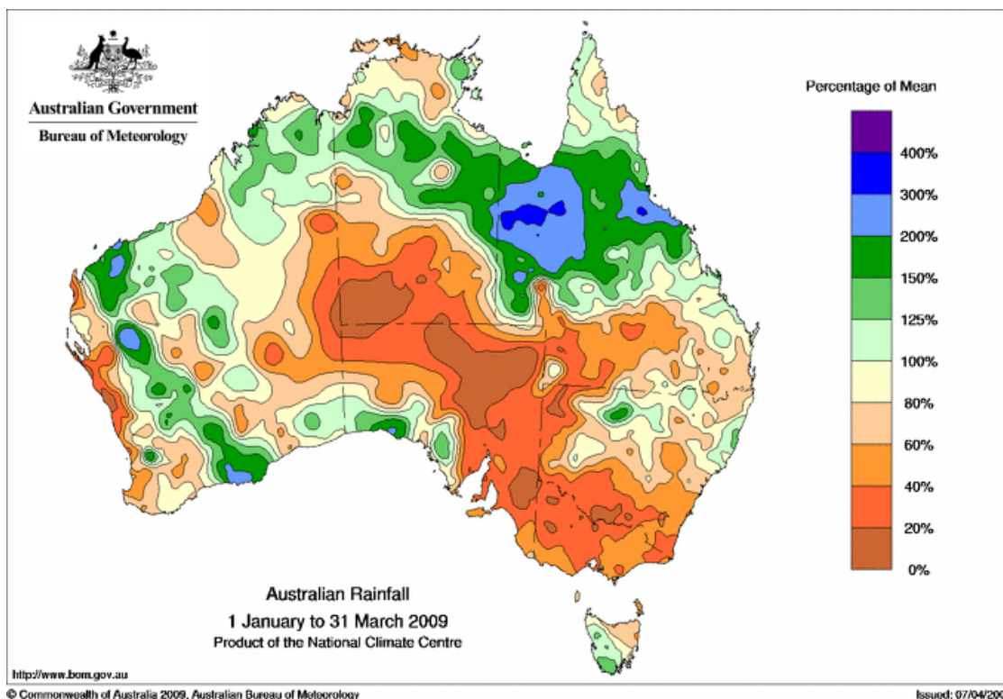
豪州 1-3月の降雨量 例年比(%) 豪州気象局
